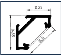
PERFIL CORNER
